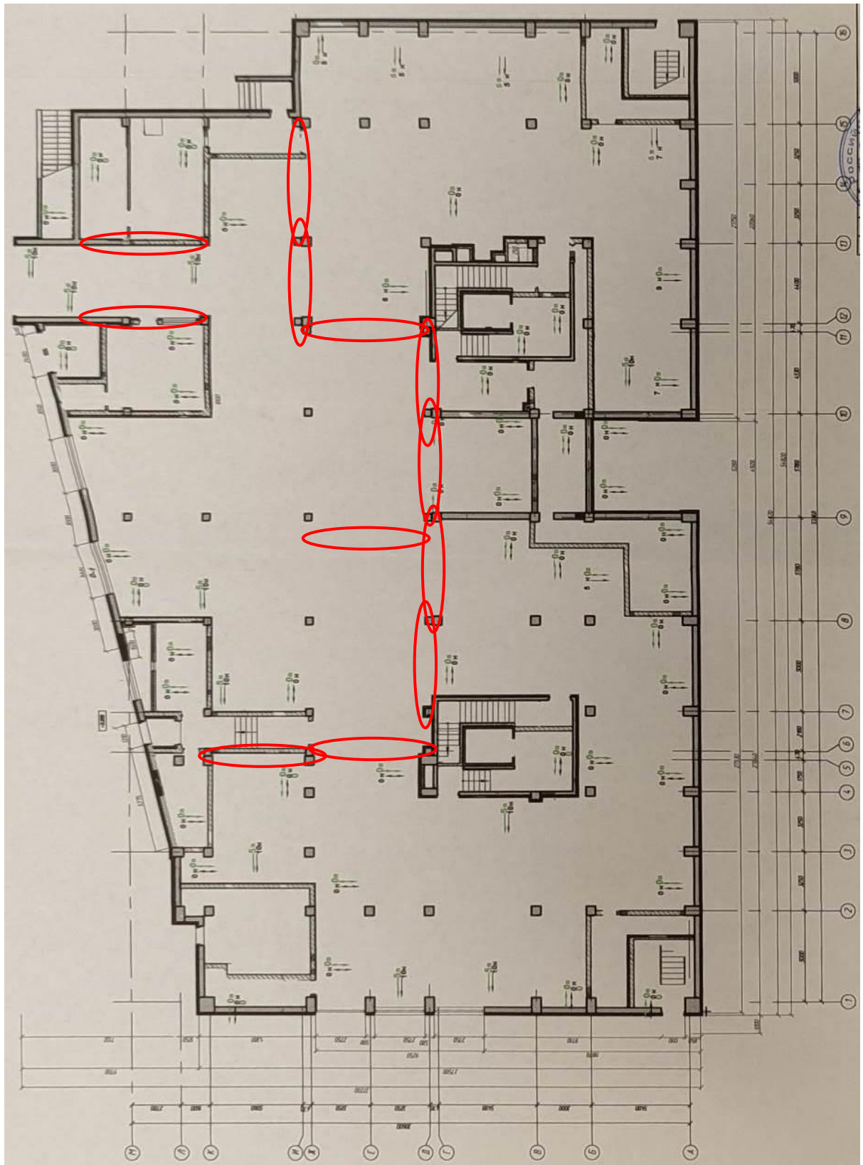
Рисунок 8. План паркинга. Карта дефектов
