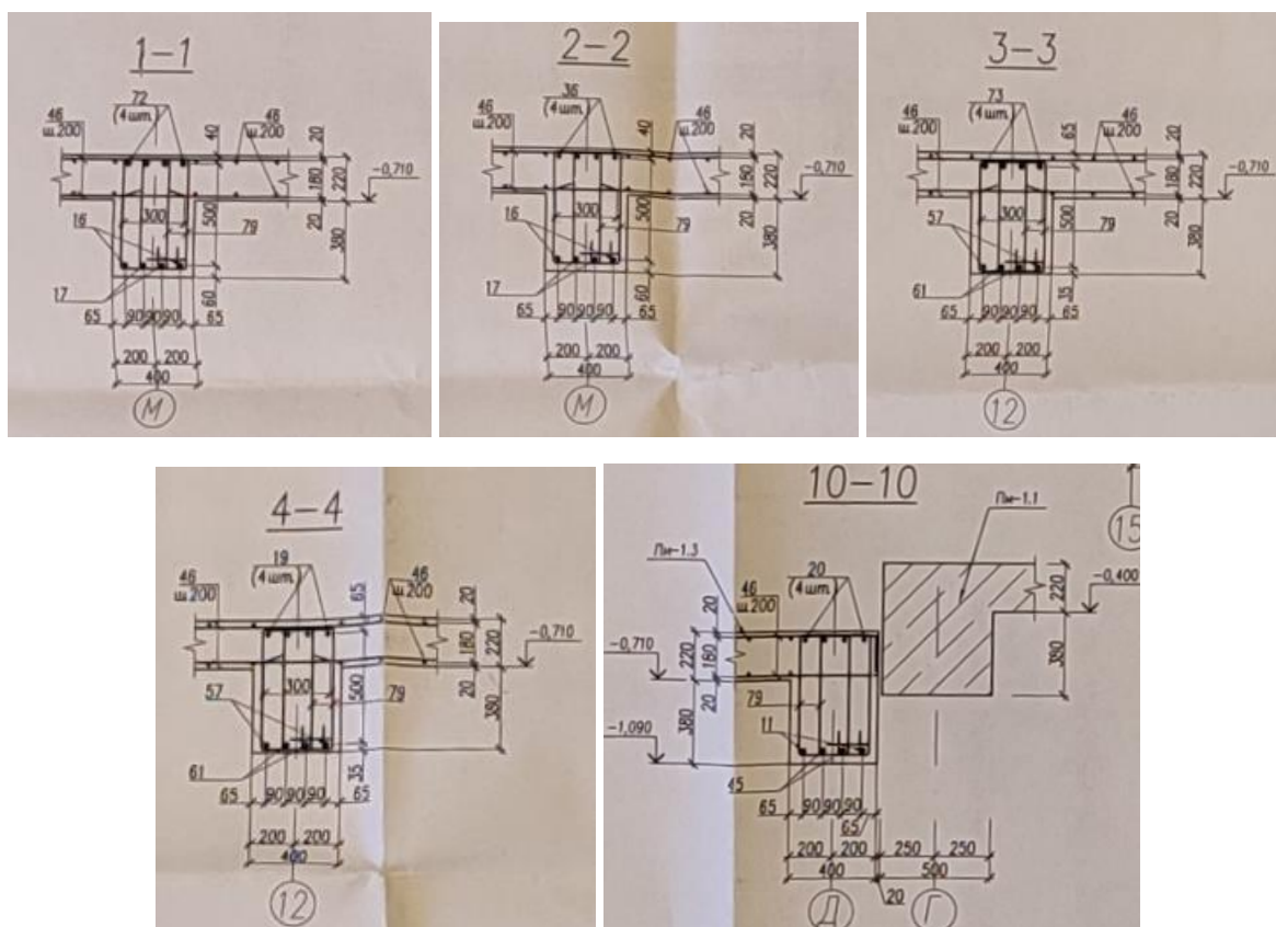
Рисунок 3, 4, 5, 6, 7. Основные сечения плиты перекрытия
