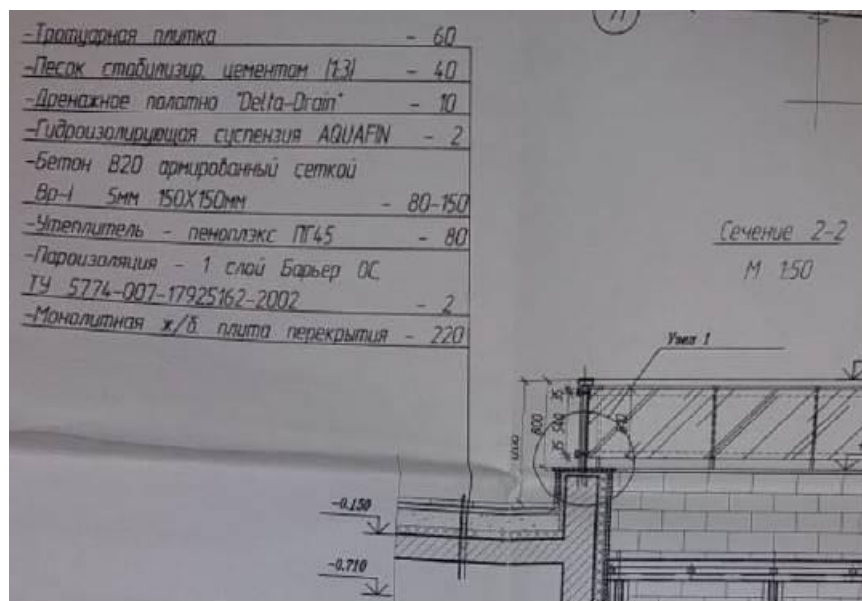
Фото 9. Состав покрытия паркинга
